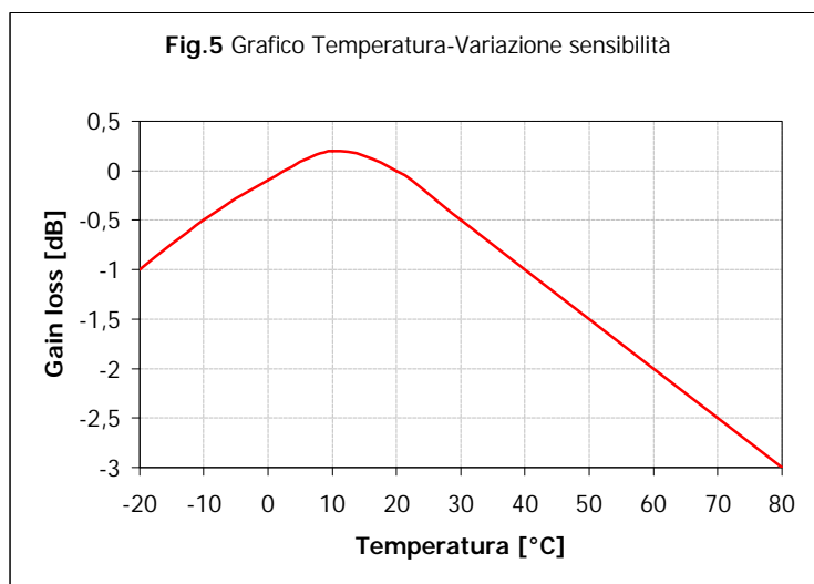
Alimentazione 5V, ingresso RF 433,92MHz, -94dBm
